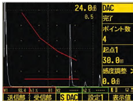
S-DAC 距離振幅特性曲線
